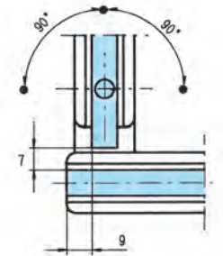
Hoja móvil
