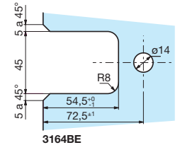
Hoja móvil
